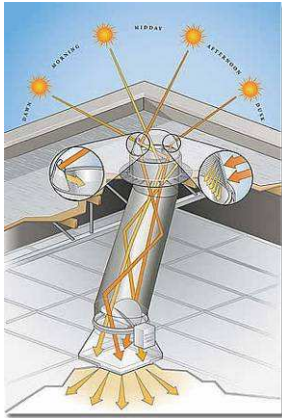
Figura 5 Pozo de luz al interior de los despachos y reducción de la demanda energética de iluminación entre los diversos edificios de referencia y LUCIA.
