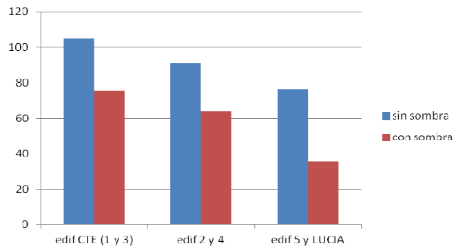
Cuadro 2. Reducción de la demanda de refrigeración en kWh/m2año con el efecto de autosombreamiento entre los diversos edificios de referencia y LUCIA
