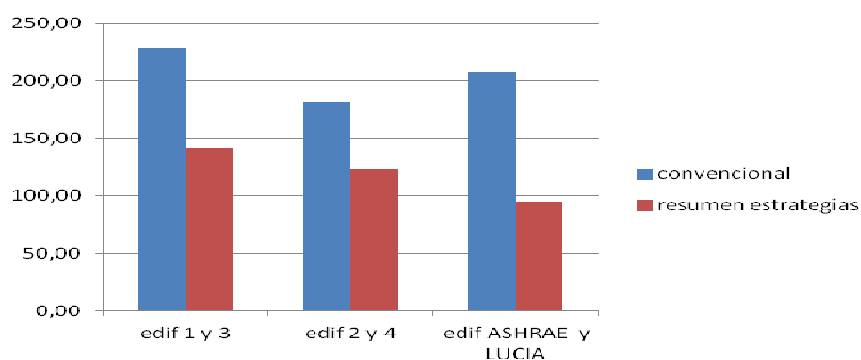
Cuadro 6. Comparativa de la reducción de la demanda total en kWh/m2año entre los diversos edificios y métodos de de referencia y el edificio LUCIA
