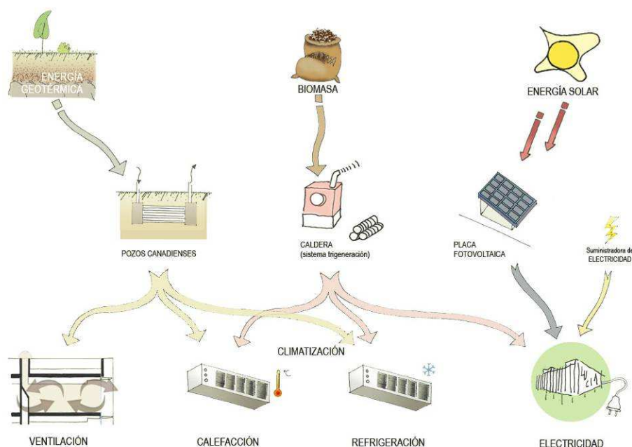
Figura 7: Esquema de integración de energías renovables (100%) en el edificio LUCIA
