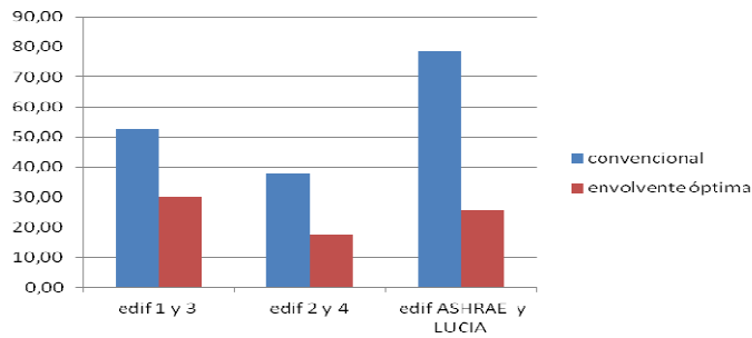
Cuadro 4. Comparativa de la reducción de la demanda de calefacción en kWh/m 2 año con las mejoras en la envolvente entre los diversos edificios y métodos de de referencia y el edificio LUCIA
