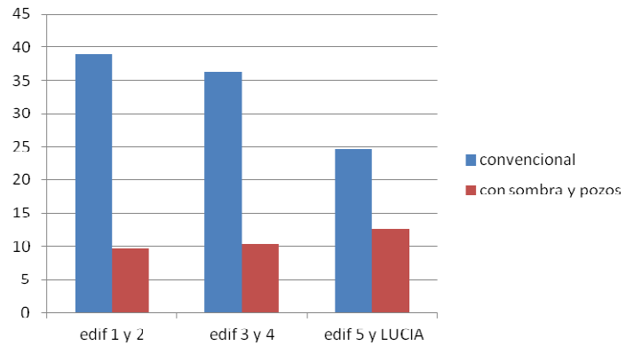
Figura 5 Pozo de luz al interior de los despachos y reducción de la demanda energética de iluminación entre los diversos edificios de referencia y LUCIA.
